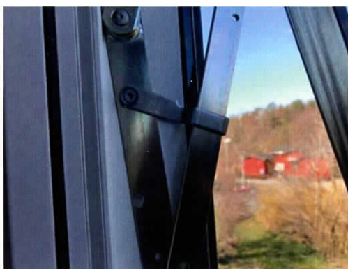
"Extra" putsbeslag i spärrat läge
